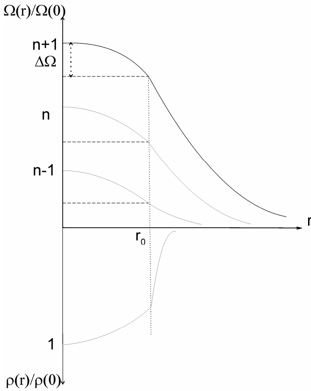
Рис. 4. Распределение по радиусу плотности заряда (внизу) и соответствующая ему угловая скорость вращения смерча (вверху) в разных квантовых состояниях (схема). Отмечена ширина зоны излучения на уровне n+1 .
