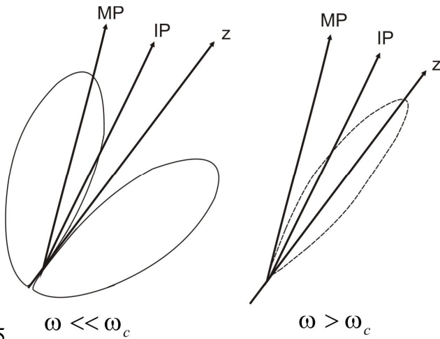
Рис. 5 \omega \ll \omega_c
